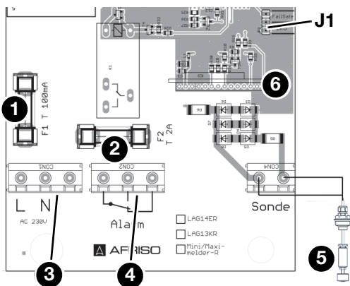
Ilustracja 5: Przyłącze elektryczne
