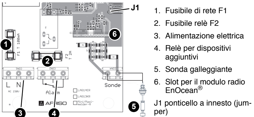
Figura 5: Allacciamento elettrico
