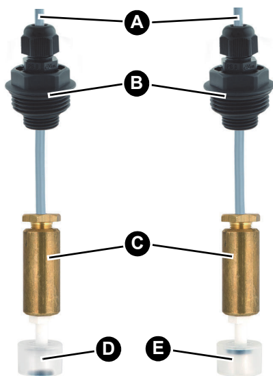
Figura 1: Sonda galleggiante
