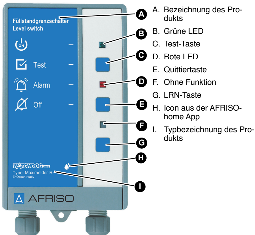
Abbildung 2: Signalteil
