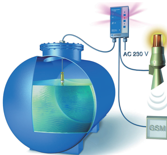
Abbildung 4: Standardanwendung Maximelder-R
