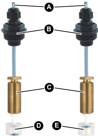
Abbildung 1: Schwimmersonde
